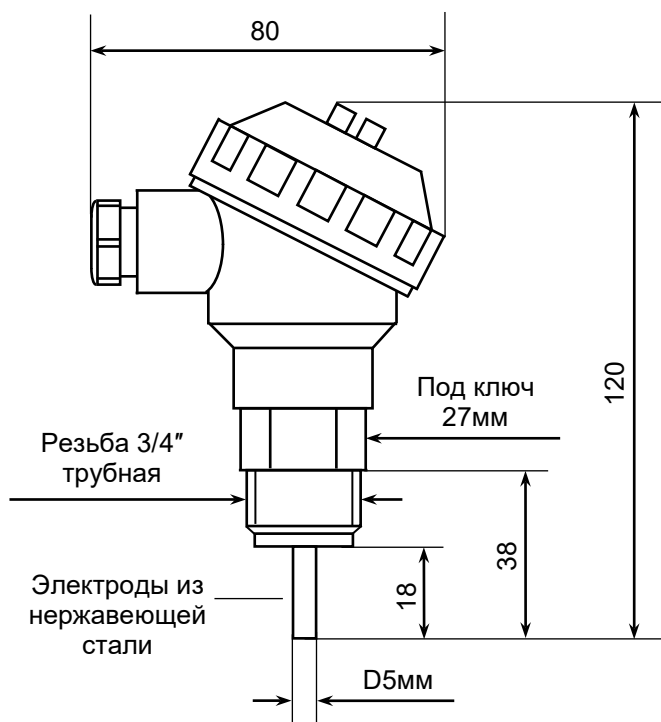
Датчик WA02-A
