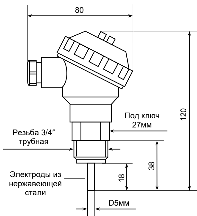
Датчик WD02
